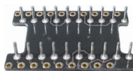
端子挿入からハンダ付け
